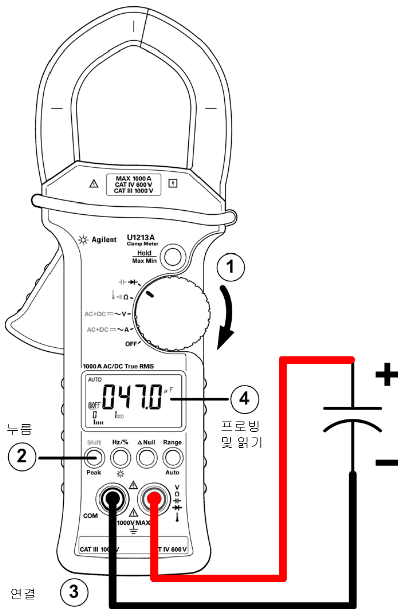
그림 2-7 캐패시턴스 측정
