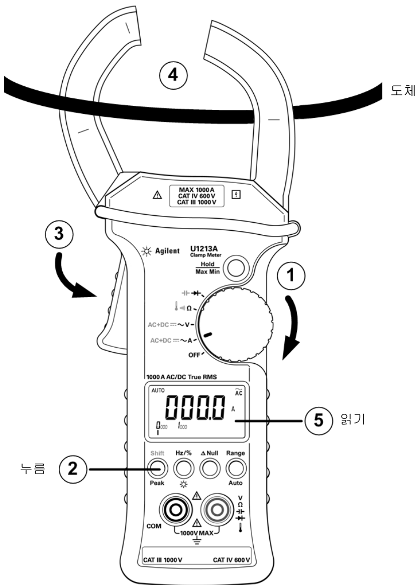
그림 2-1 전류 측정
