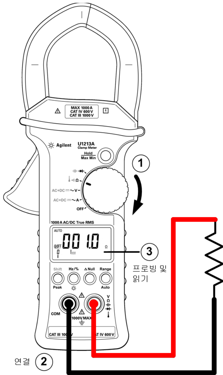
그림 2-3 저항 측정
