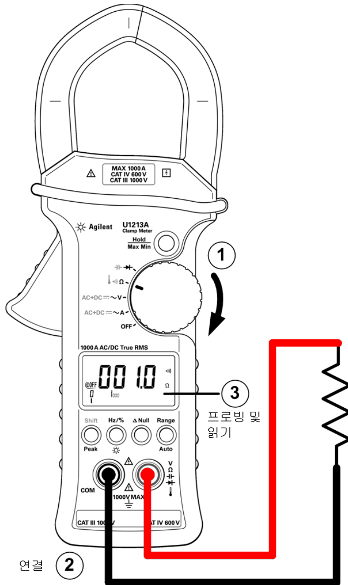
그림 2-4 연속성 테스트
